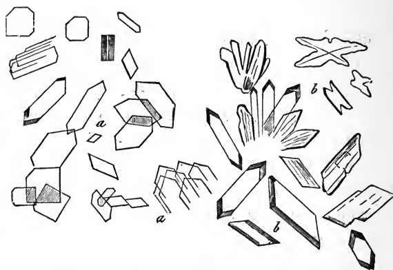
Fig. 9.— a , UREA NITRATE; b , UREA OXALATE.
